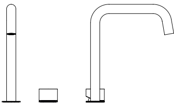
2-Loch Waschtischarmaturen. 2-hole basin mixer – 2x Ø 39,6 x 212 x 180 mm
