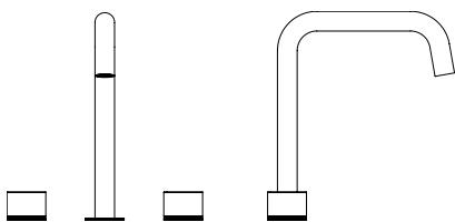
3-Loch Waschtischarmaturen. 2-hole basin mixer – 3x 39,6 x 212 x 180 mm
